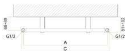
CONEXIÓN LATERAL
