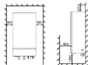
Espacio instalación
