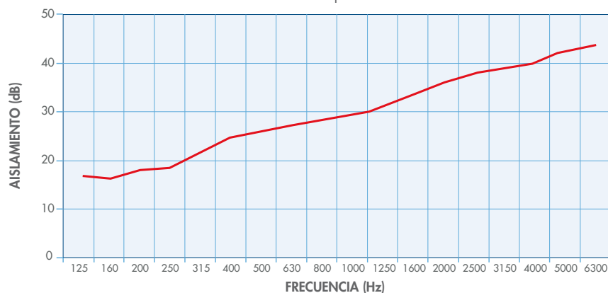
TRANSMISSION LOSS (DIN 52210) masa de espesor 2 mm
