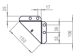
DETALLE A
