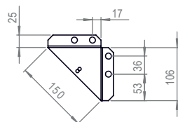
DETALLE A
