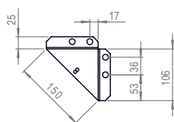
DETALLE A
